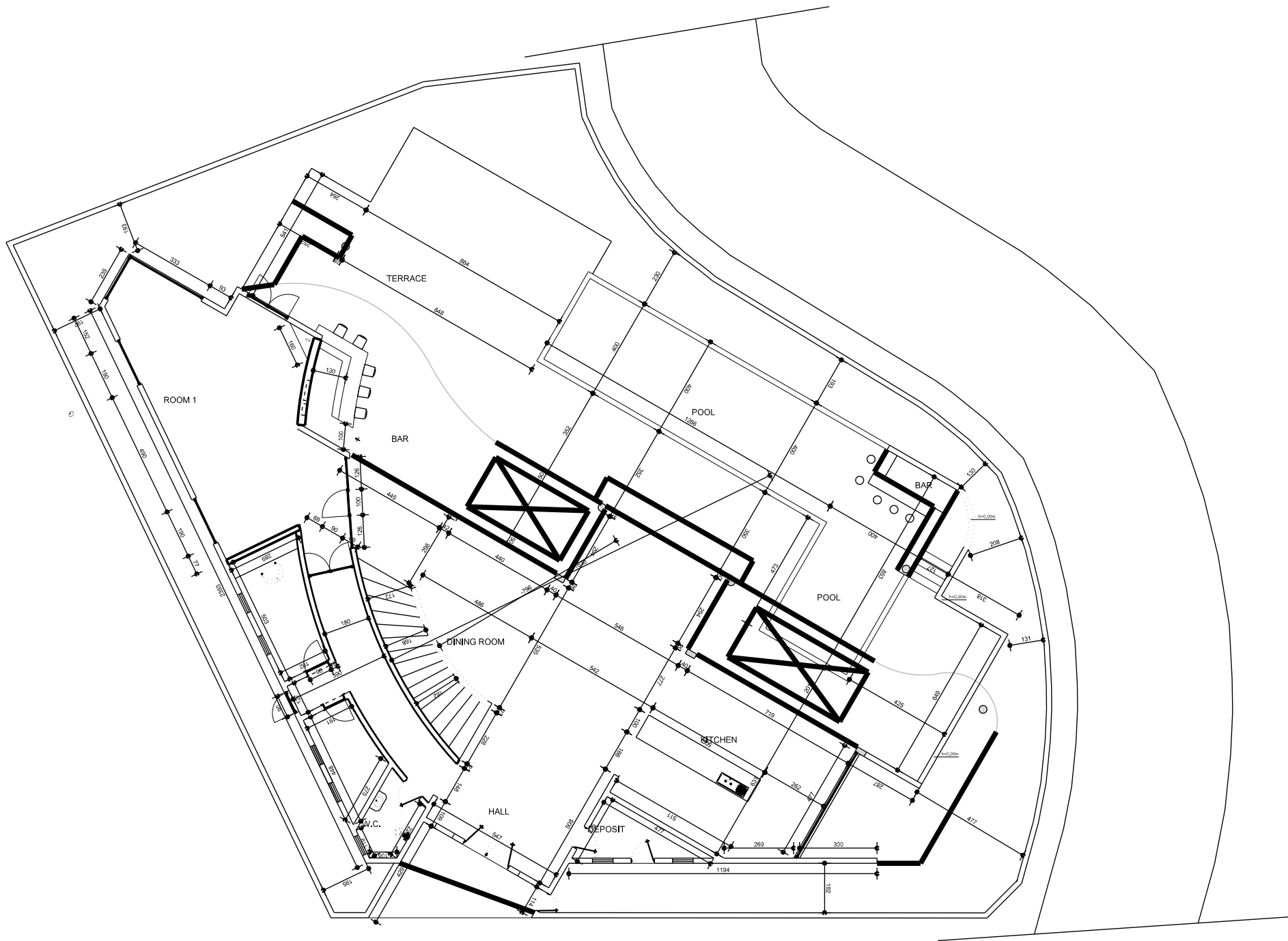
Planta Dimensionada Nivel 0
