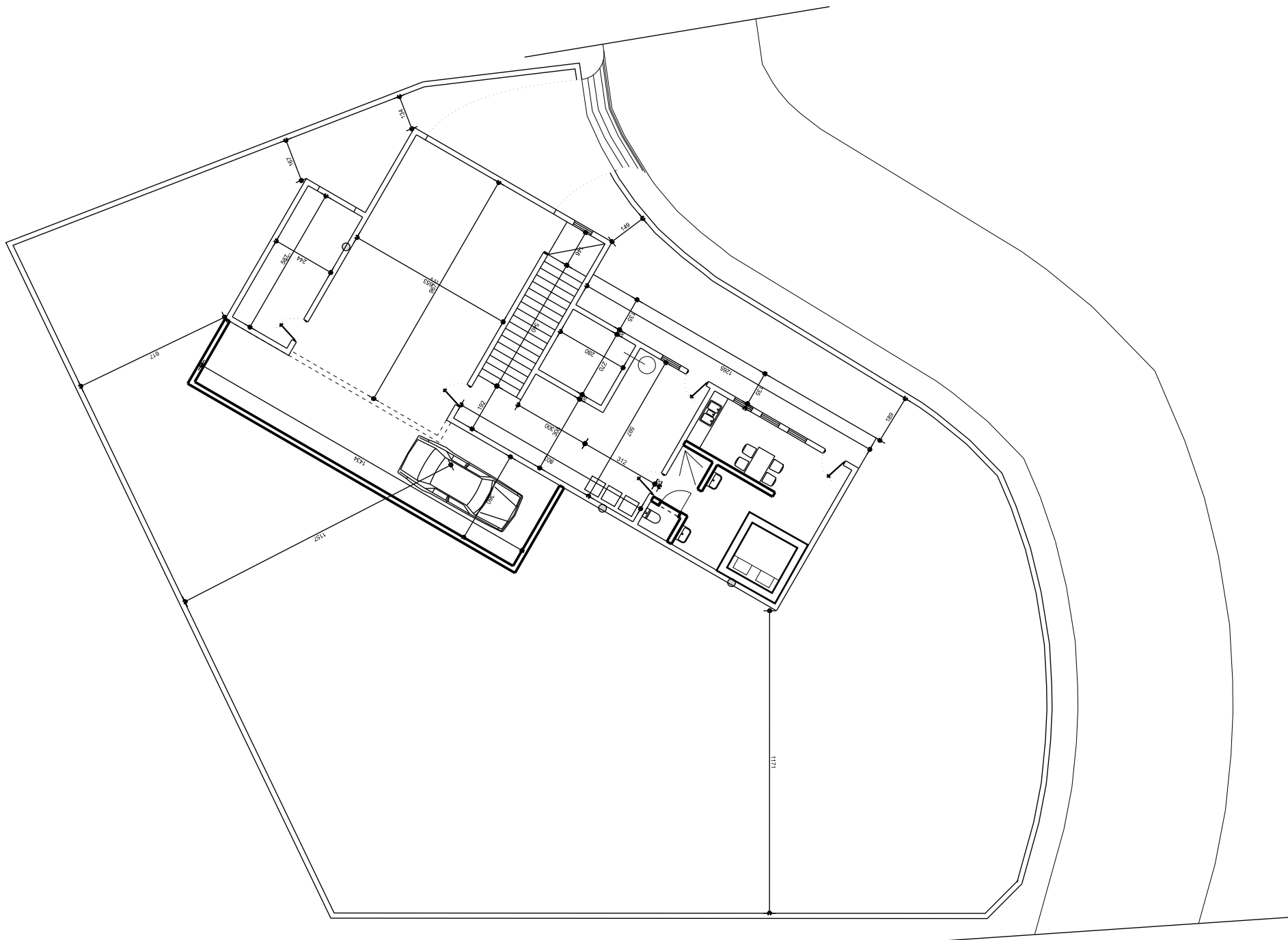
Planta Dimensionada Nivel-2
