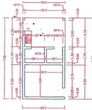
PLANTA DIMENSIONADA AREA DE SERVIDIO Esc: 1:100
