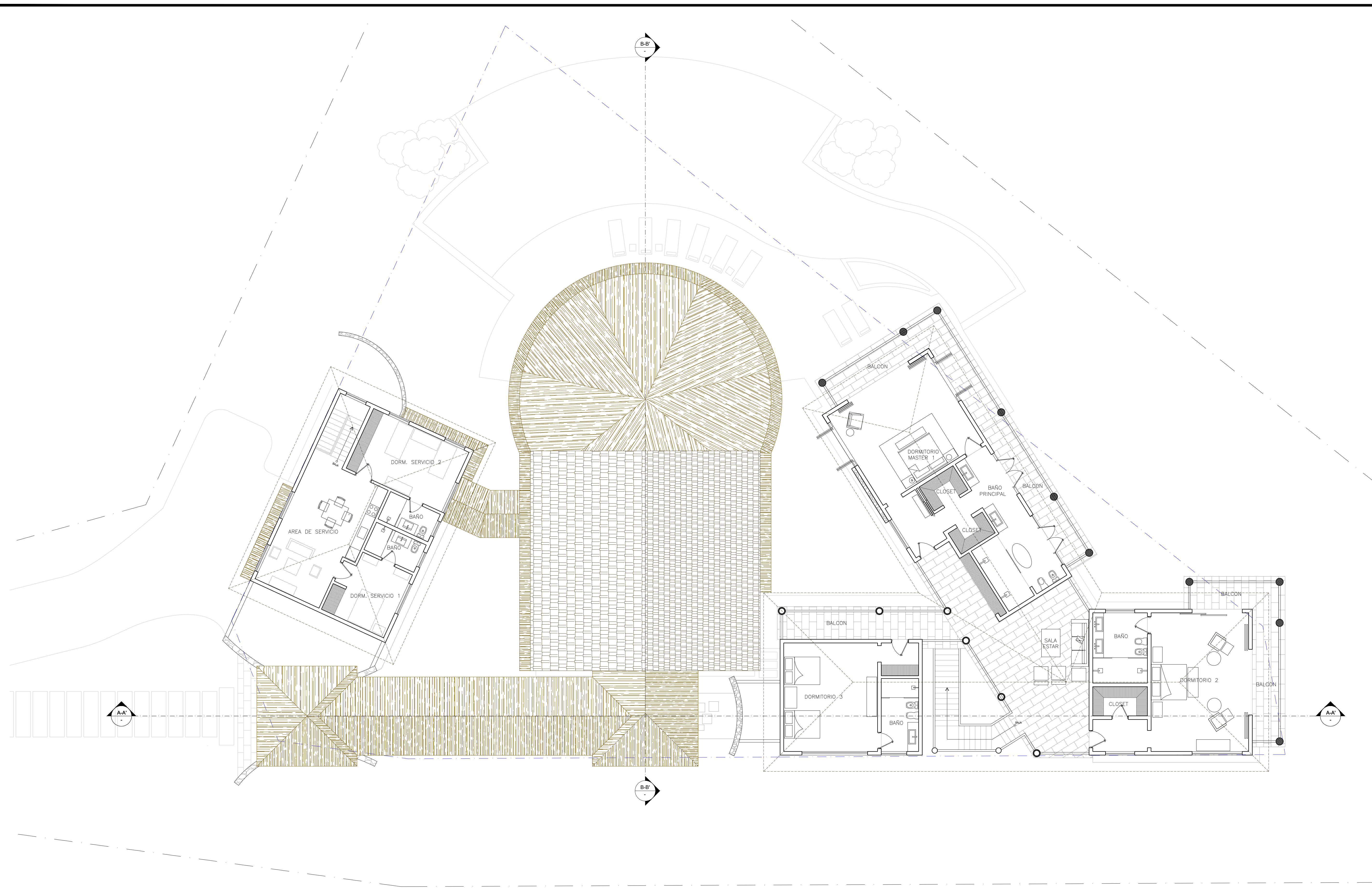
PLANTA ARQUITECTONICA 2DO NIVEL ESC. 1:100
